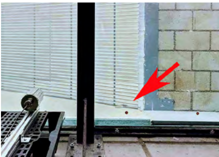
Bild 3: Eine Kamera erfasst im VAW-Labor an der ETH Zürich das Verhalten von Fischen am Leitrechen. Rechts unten am Rechen (mit Pfeil markiert) ist eine Barbe zu sehen, die gegen das von links anströmende Wasser schwimmt und durch die horizontalen Stäbe des Rechens zu schlüpfen droht (Foto: VAW).
