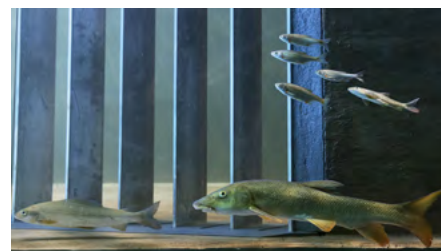
Bild 10: Barben (unten) und Schneider (oben rechts) schwimmen an einem Fischleitrechen im Labor (Foto: VAW).
