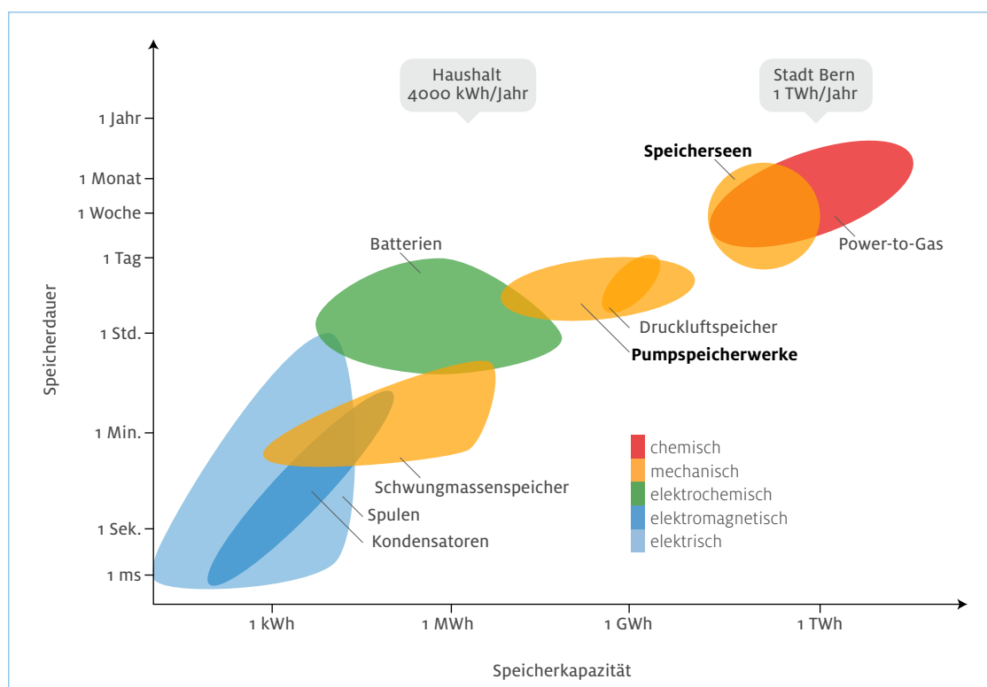
Speicherarten im Vergleich nach Speicherkapazität und Speicherdauer (Quelle [bearbeitet]: M. Sterner: Energiespeicher – Bedarf, Technologien, Integration; Springer Verlag 2017)
